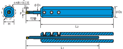
小徑內孔車刀架 Mini Boring Bar
