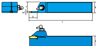
外徑切斷刀架 External Grooving
