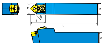
外徑車刀架 Tool holder
