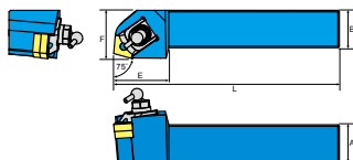
外徑車刀架 Tool holder
