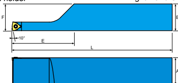
本圖所示為右手刀 (R) Right-Hand Show
