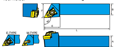
外徑車刀架 Tool holder
