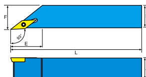
外徑車刀架 Tool holder
