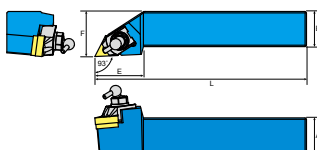
外徑車刀架 Tool holder
