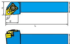
本圖所示為右手刀 (R) Right-Hand Show
