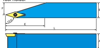
外徑車刀架 Tool holder
