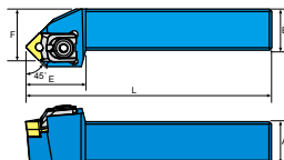
本圖所示為右手刀 (R) Right-Hand Show
