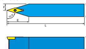
外徑車刀架 Tool holder
