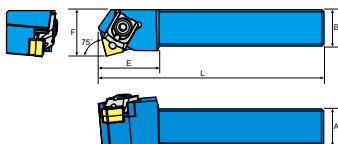
外徑車刀架 Tool holder
