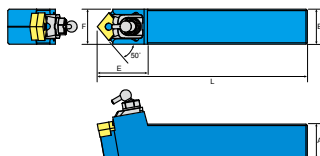
外徑車刀架 Tool holder
