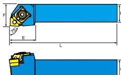
本圖所示為右手刀 (R) Right-Hand Show
