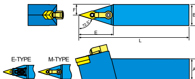
外徑車刀架 Tool holder
