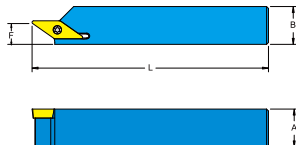
外徑車刀架 Tool holder
