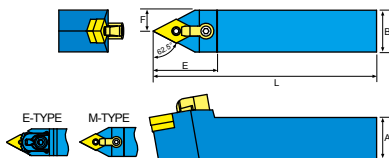
外徑車刀架 Tool holder
