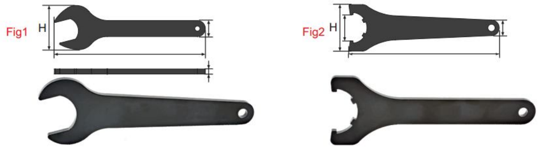
寸法 Dimension(mm)
