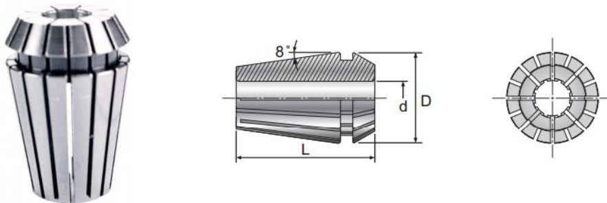
寸法 Dimension(mm)
