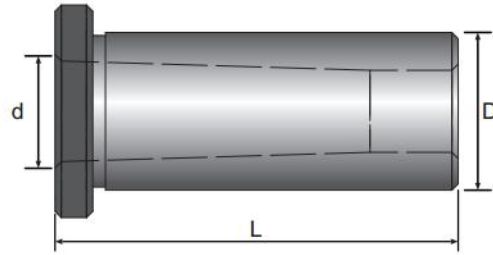
寸法 Dimension(mm)
