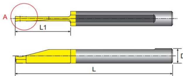
寸法 Dimension(mm)
