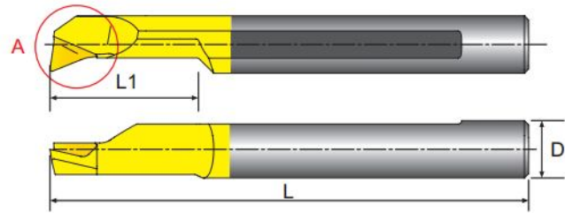
寸法 Dimension(mm)
