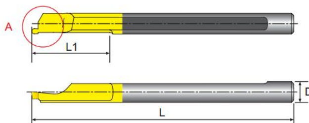
寸法 Dimension(mm)
