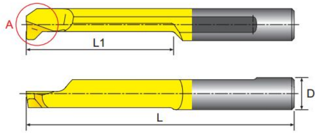
寸法 Dimension(mm)
