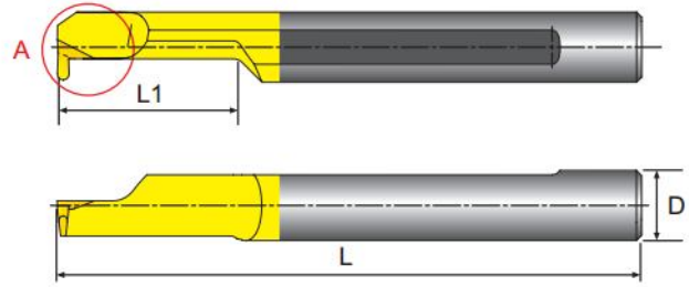
寸法 Dimension(mm)
