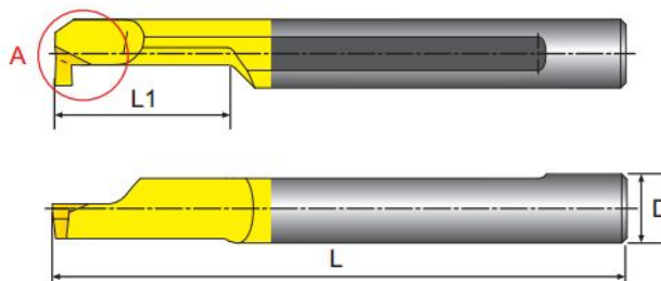
寸法 Dimension(mm)
