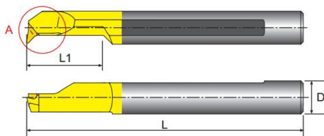
寸法 Dimension(mm)
