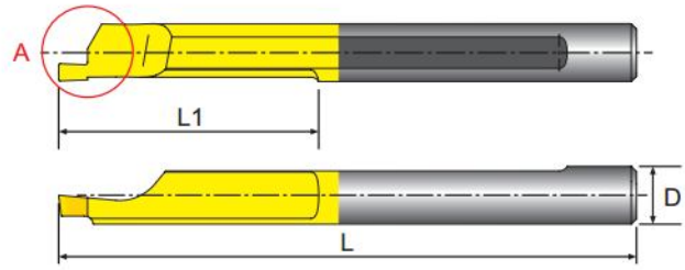
寸法 Dimension(mm)
