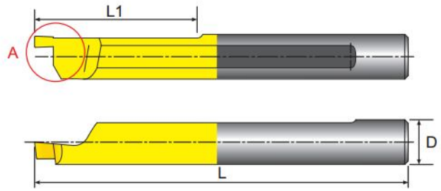
寸法 Dimension(mm)
