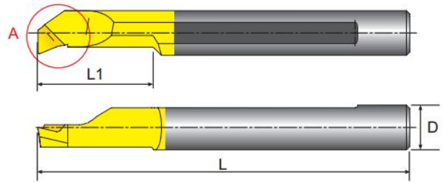
寸法 Dimension(mm)
