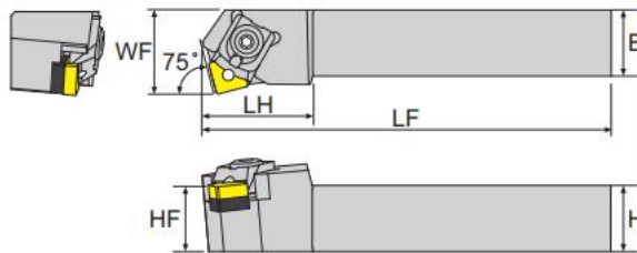
寸法 Dimension(mm)
