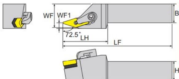
寸法 Dimension(mm)
