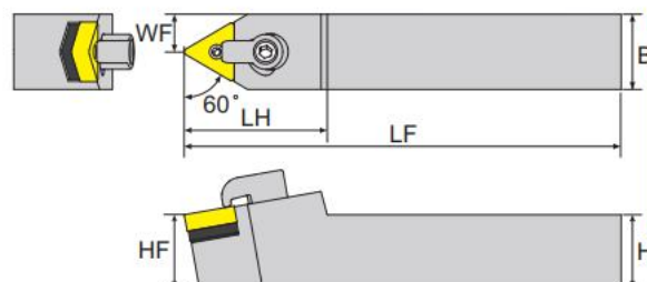
寸法 Dimension(mm)
