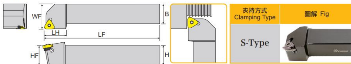
寸法 Dimension(mm)
