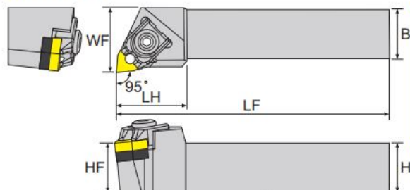
寸法 Dimension(mm)
