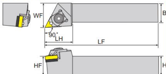
寸法 Dimension(mm)
