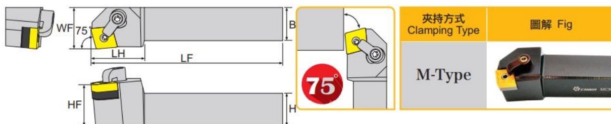
寸法 Dimension(mm)
