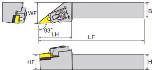
寸法 Dimension(mm)
