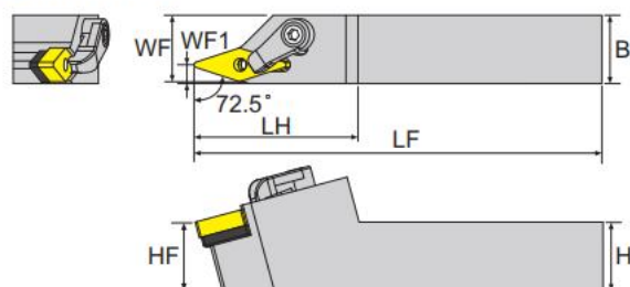
寸法 Dimension(mm)
