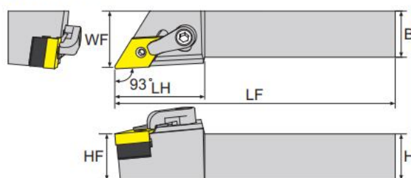
寸法 Dimension(mm)
