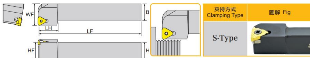
寸法 Dimension(mm)
