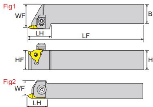
寸法 Dimension(mm)
