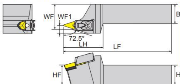
寸法 Dimension(mm)
