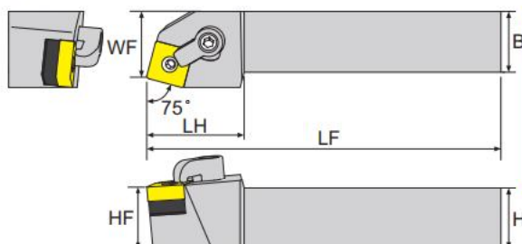
寸法 Dimension(mm)
