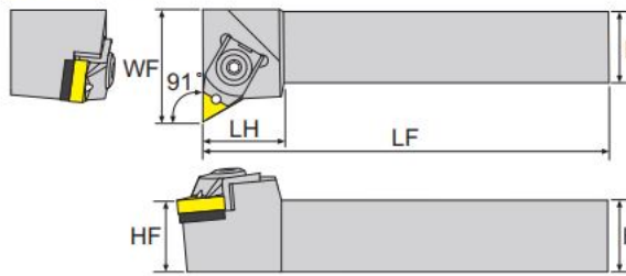
寸法 Dimension(mm)
