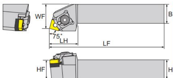
寸法 Dimension(mm)
