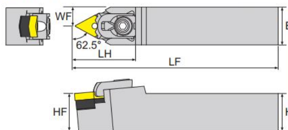
寸法 Dimension(mm)
