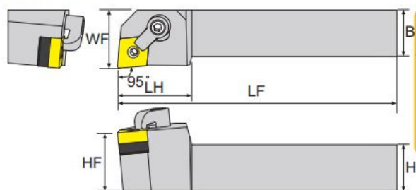
寸法 Dimension(mm)
