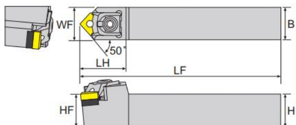
寸法 Dimension(mm)
