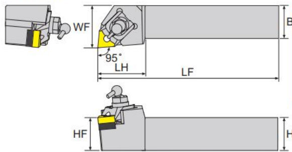
寸法 Dimension(mm)
