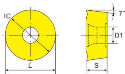
塗層硬質合金 Carbide Coated
