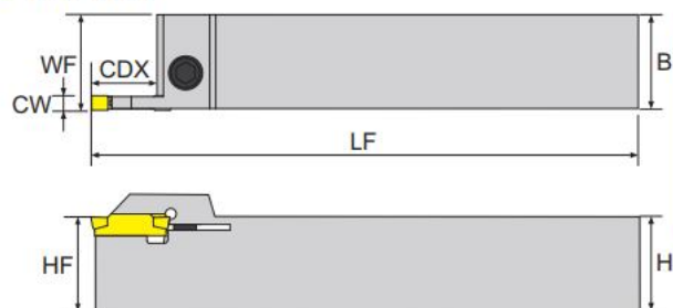
EDGH 外徑切斷刀架 EDGH External Grooving
