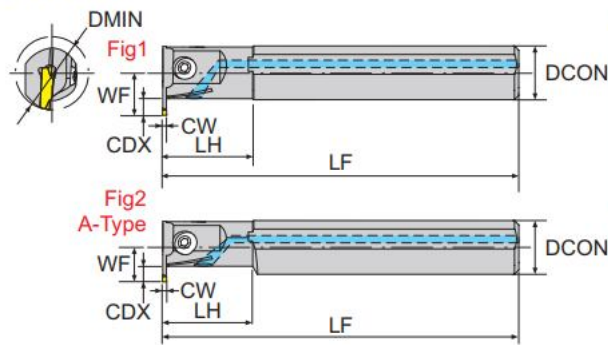
HOZ 內徑開槽刀架 HOZ Internal Grooving
