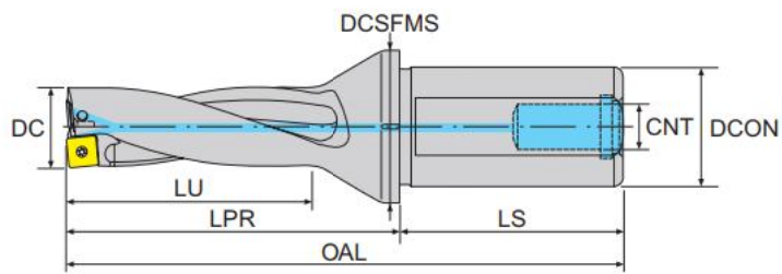
寸法 Dimension(mm)
