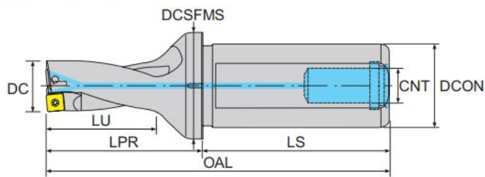
寸法 Dimension(mm)
