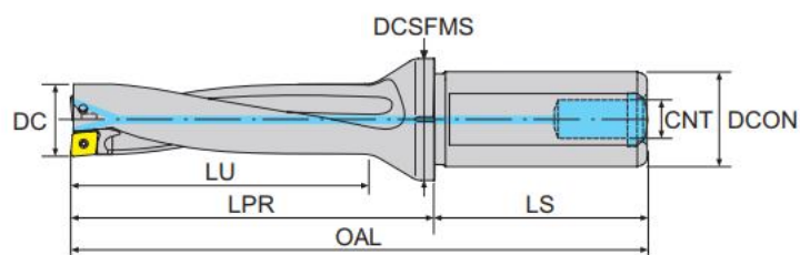
寸法 Dimension(mm)
