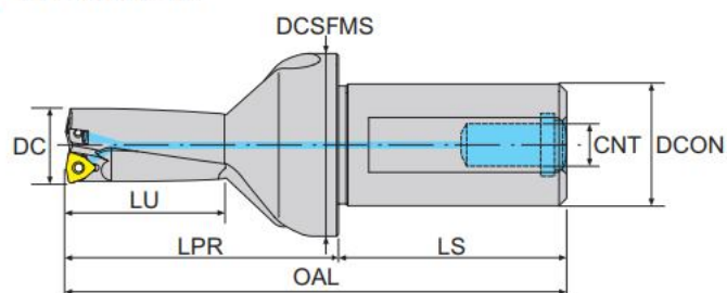
寸法 Dimension(mm)
