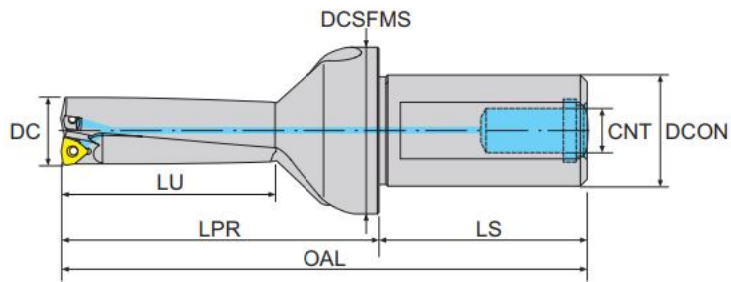
寸法 Dimension(mm)
