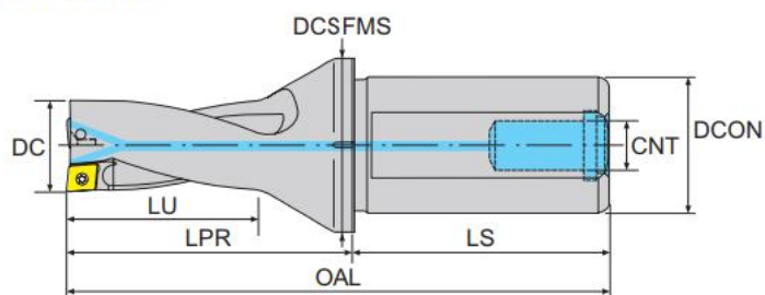
寸法 Dimension(mm)
