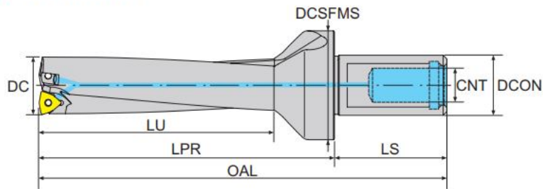
寸法 Dimension(mm)
