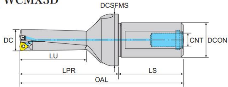
寸法 Dimension(mm)
