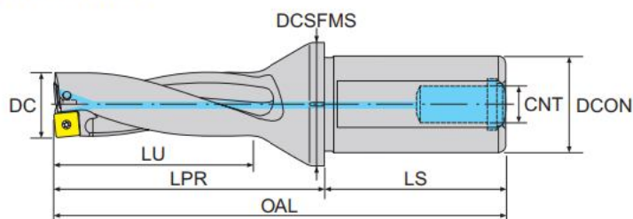
寸法 Dimension(mm)
