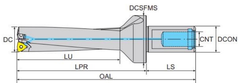
寸法 Dimension(mm)
