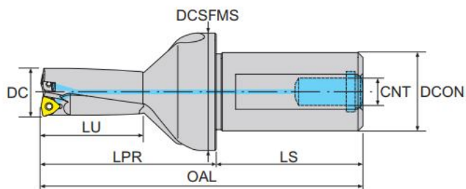
寸法 Dimension(mm)
