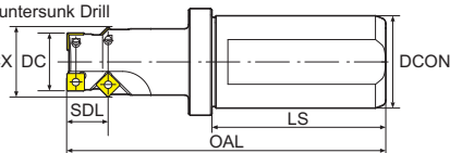
沉頭鑽頭範例： Countersunk Drill
