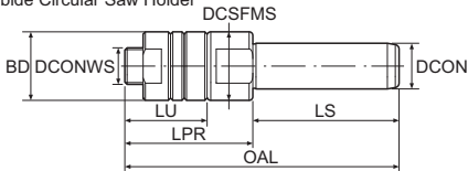
圓型鋸片刀桿範例： Carbide Circular Saw Holder
