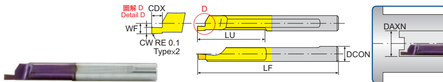
微小徑端面鑄鋼內徑車刀 Tiny Grooving Carbide Boring Bar
