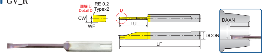
微小徑端面切槽鎢鋼內徑車刀 Tiny Face Grooving Carbide Boring Bar
