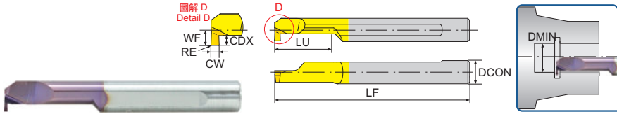
微小徑開槽鎢鋼內徑車刀 Tiny Grooving Carbide Boring Bar
