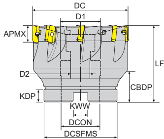
寸法 Dimension(mm)
