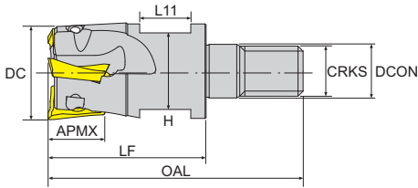
寸法 Dimension(mm)
