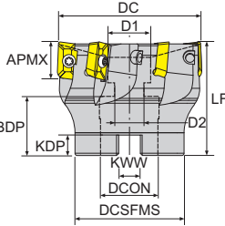
寸法 Dimension(mm)
