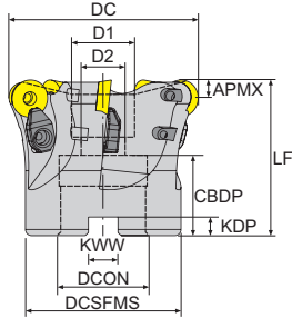
寸法 Dimension(mm)
