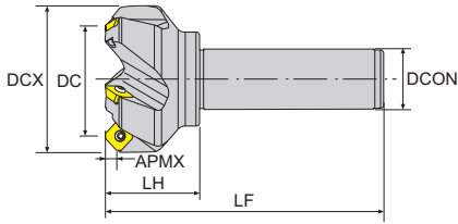
寸法 Dimension(mm)
