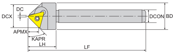
寸法 Dimension(mm)
